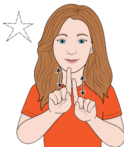
star
