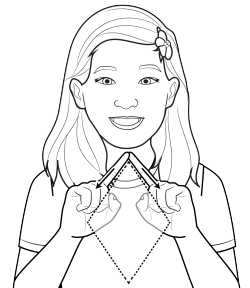
rhombus
